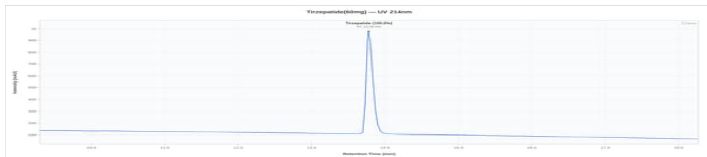
Tirzepatide 60mg - 2026-002: UV Chromatogram
